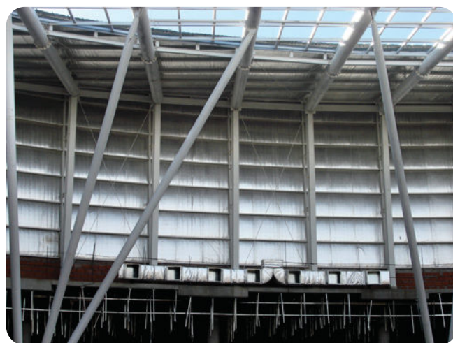
Utilización Filtro Tensado Alu en cubierta y cerramiento vertical.
